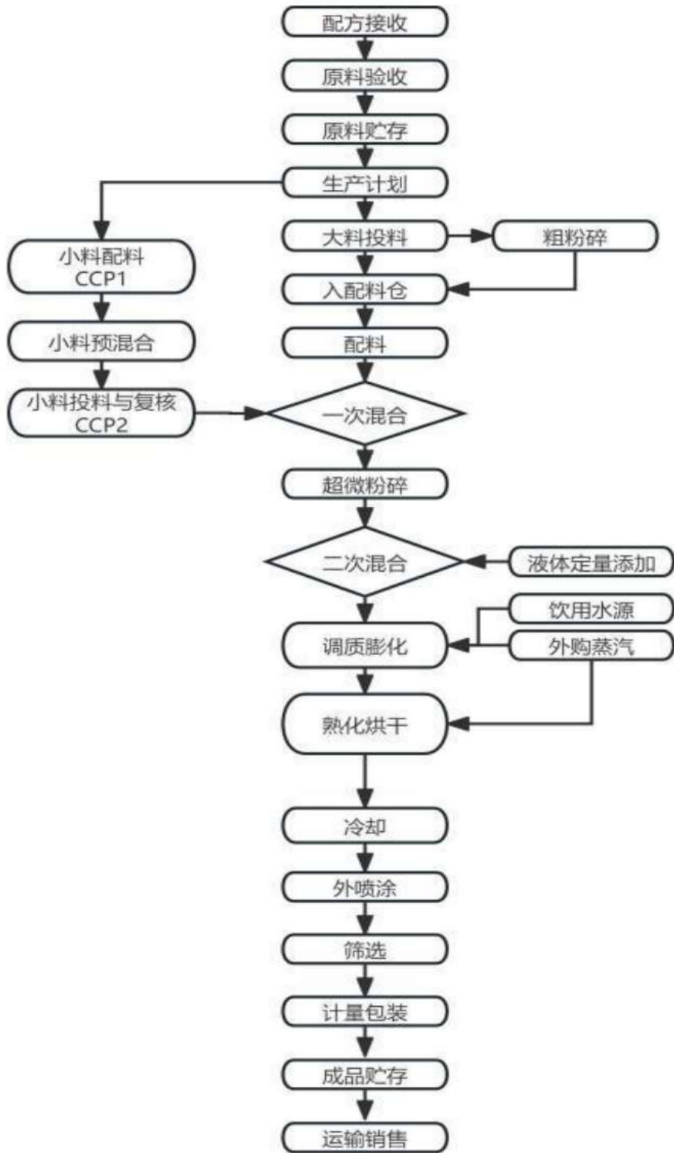
图 3-1 受核查方生产工艺流程图
